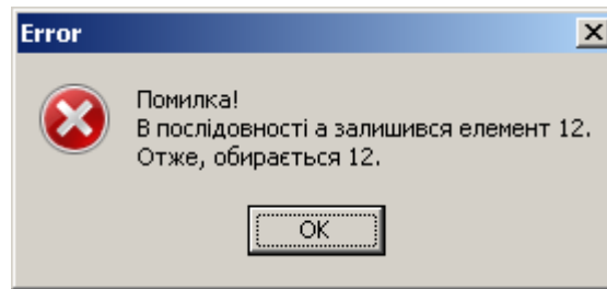
Рисунок 4.24 – Пояснення помилки
