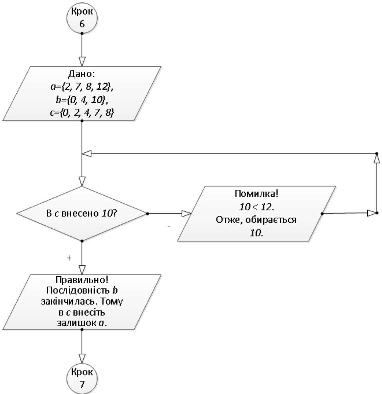
Рисунок 3.6 – Блок-схема алгоритму
