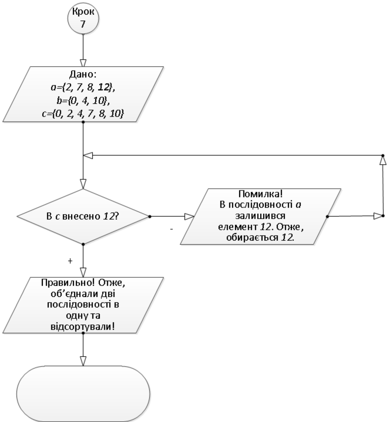
Рисунок 3.7 – Блок-схема алгоритму
