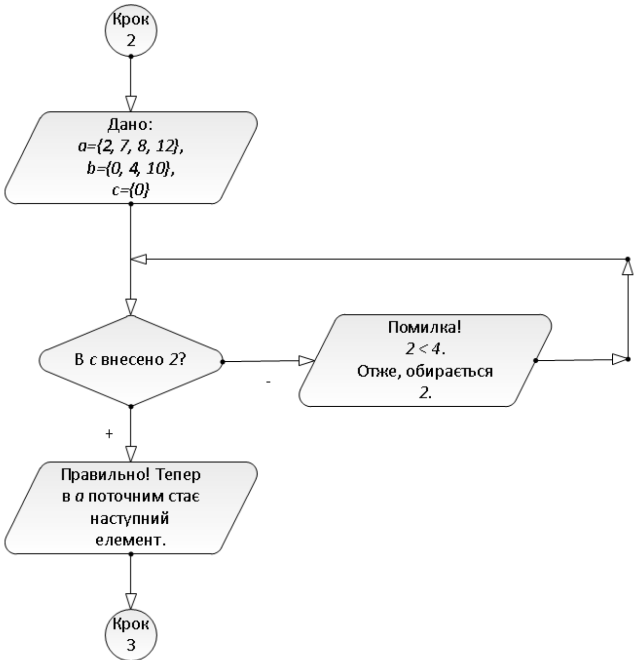
Рисунок 3.2 – Блок-схема алгоритму
