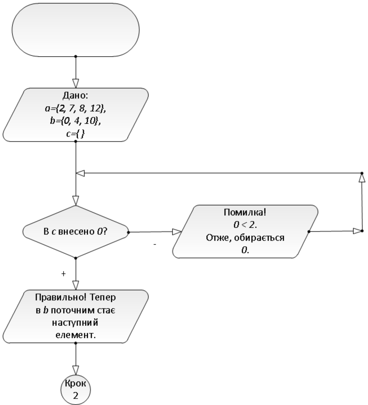
Рисунок 3.1 – Блок-схема алгоритму
