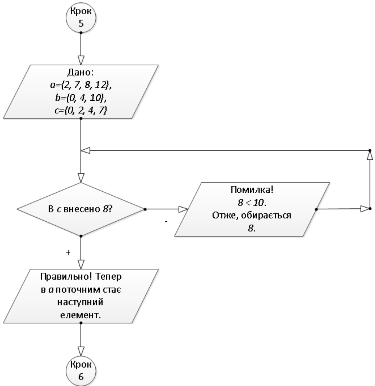
Рисунок 3.5 – Блок-схема алгоритму
