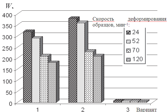
Рисунок 1 – Водопомокаемость (W) кожевенного материала в динамических условиях при разных скоростях деформирования образцов кож
